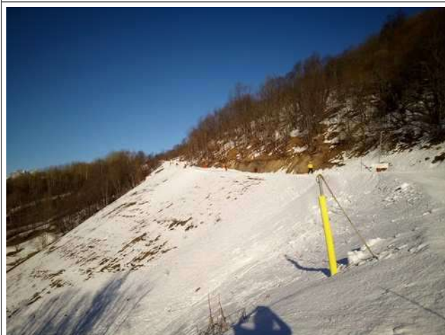
▲ La partie haute du remblai et la piste de ski vus du Sud
