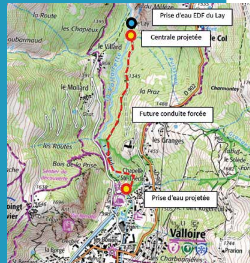
Figure 1 : Tracé du projet hydroélectrique de la Valloirette
